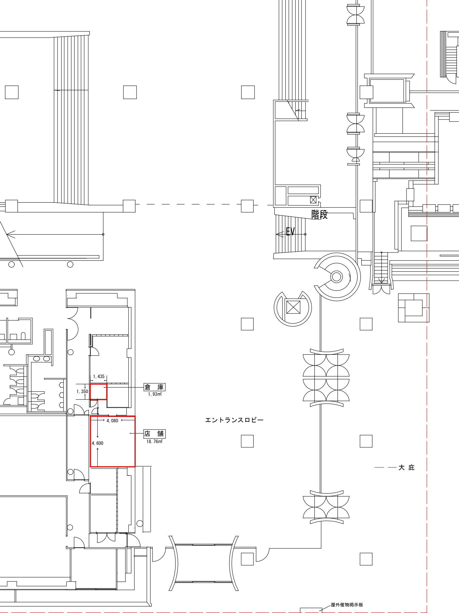
ミュージックギフトショップ 店舗平面図
